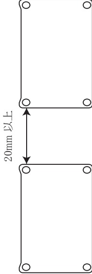
【電源間距離】
